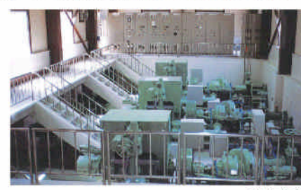
揚水機場
